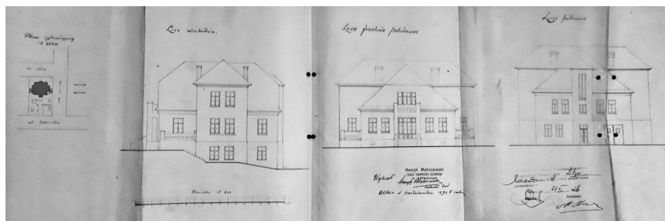
Plan domu przy Gwareckiej 15 z 21.11.1928 r. (źródło: AP Katowice, 1204/377)
