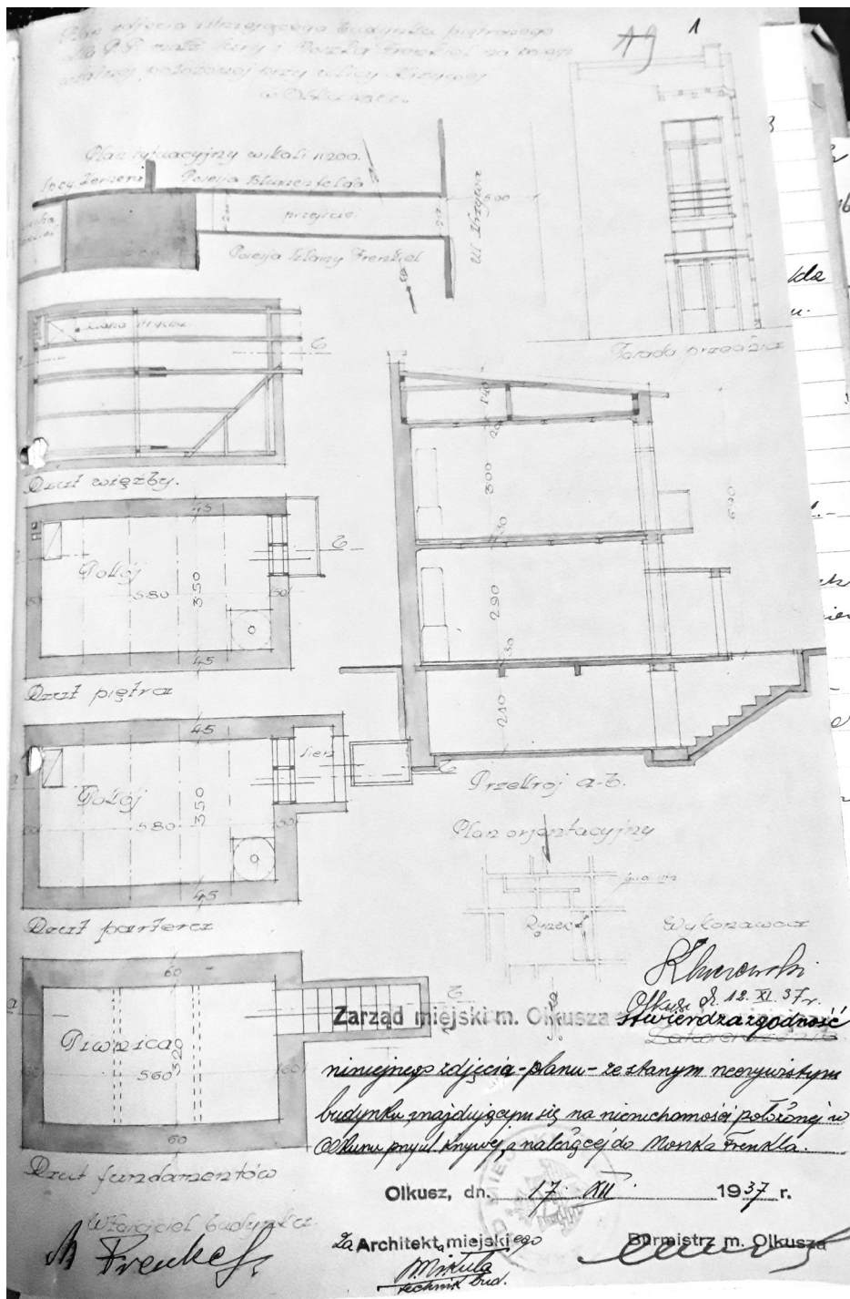
Plan budynku przy Krzywej na nieruchomości Moszka Frenkla z 17.12.1937 r. (źródło: AP Katowice, sygn. 1204/384, k. 1)
